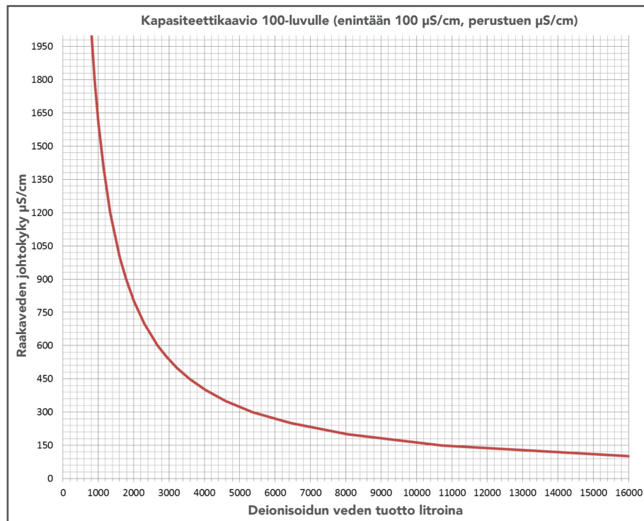
Kuva 9-9: Kaavio kapasitanssin määrittämiseksi johtokyvyn perusteella
