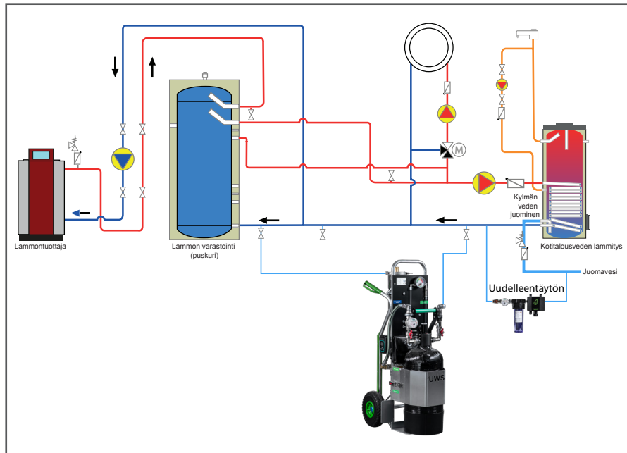
Kuva 4-4: Ohitusmenetelmän kytkentäkaavio
