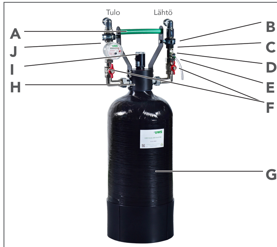
Kuva 3-2: Heaty Small 100 HW -valmisteluyksikön komponentit
