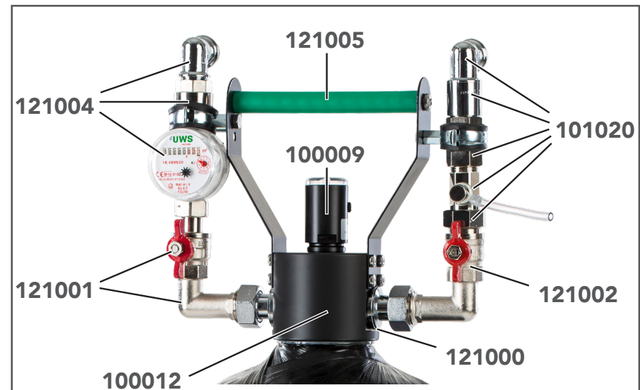
Kuva 6-8: Heaty Small 100 HW varaosat
