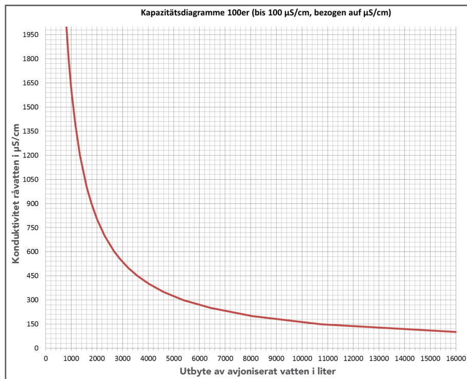
Bild 9-9: Diagram för att bestämma kapacitansen utifrån konduktiviteten
