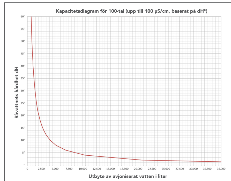
Bild 9-10: Diagram för att bestämma kapaciteten utifrån råvattnets hårdhet
