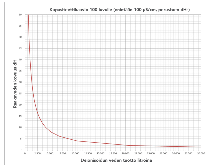
Kuva 9-10: Kaavio kapasiteetin määrittämiseksi raakaveden kovuuden perusteella
