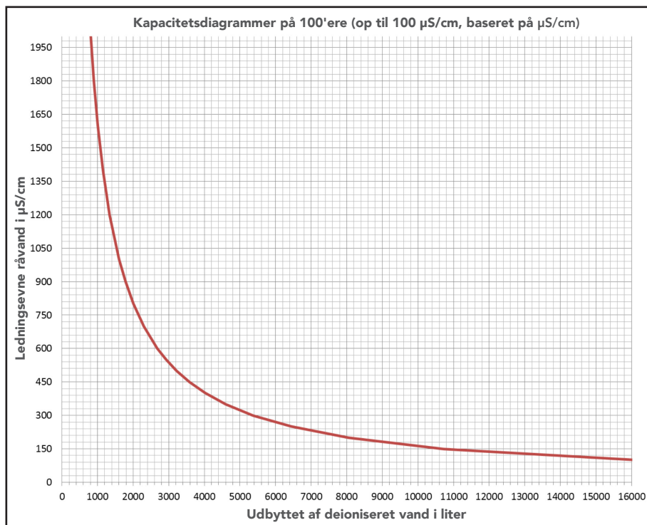
Billede 9-9: Diagram til bestemmelse af kapaciteten ud fra ledningsevnen
