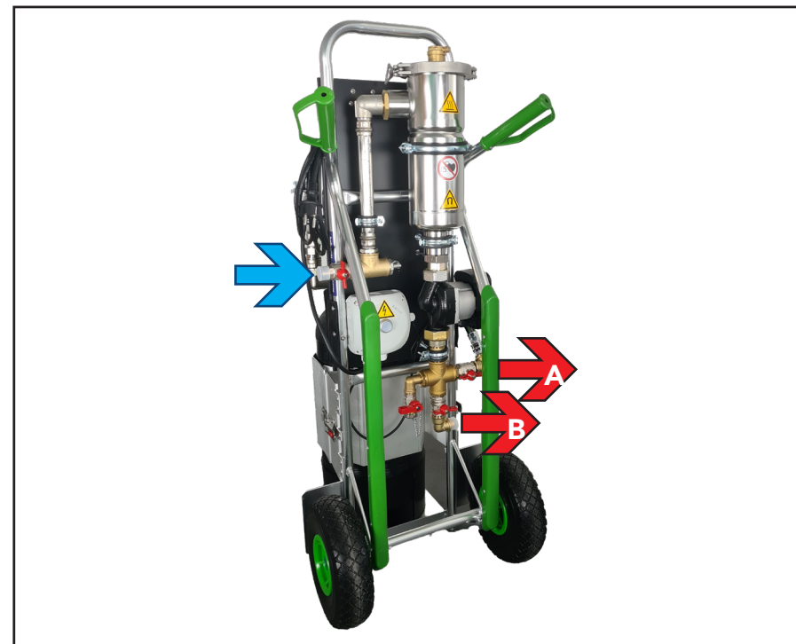
Fig. 5-5: Diagram over filtreringstilslutning
