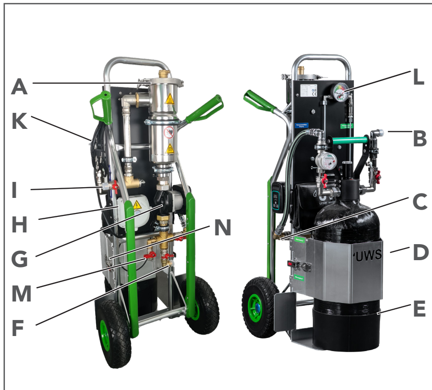
Fig. 3-1: Översikt över enhetens komponenter
