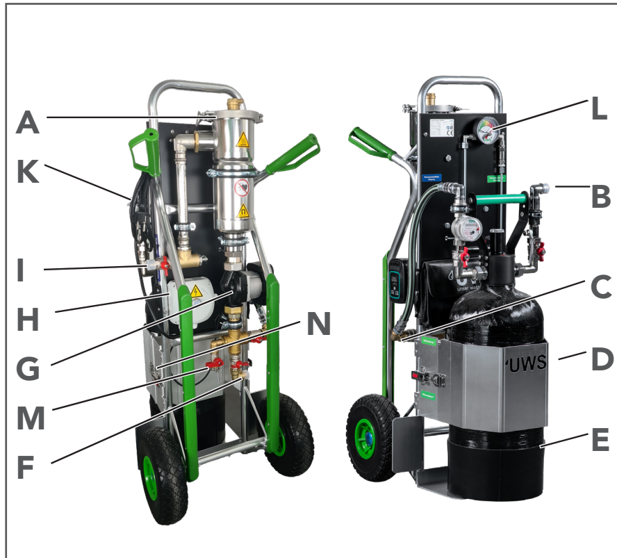
Kuva 3-1: Laitteen komponenttien yleiskatsaus
