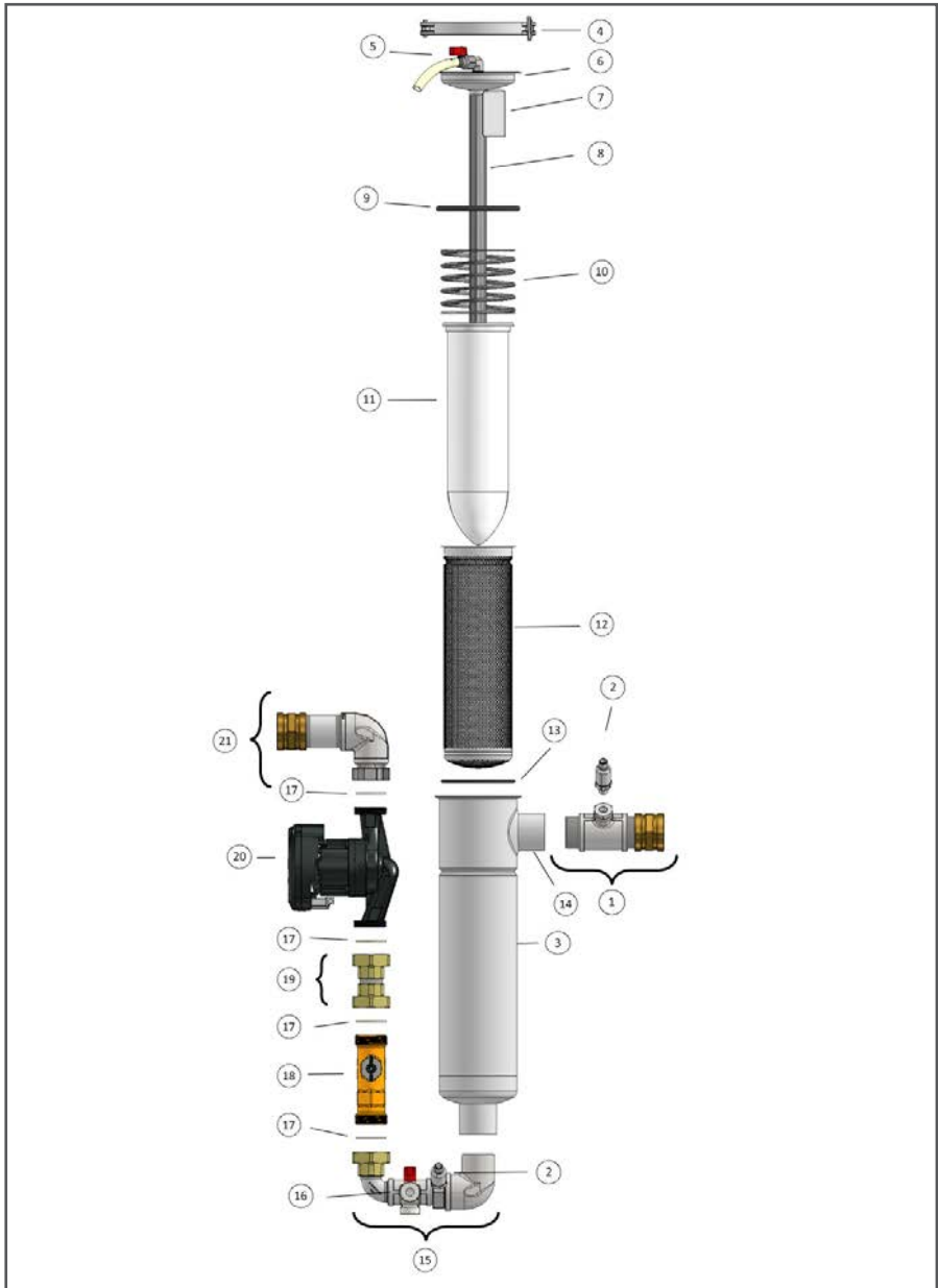
Bild 6-4: Ersatzteile MAGella Side Stream Filter
