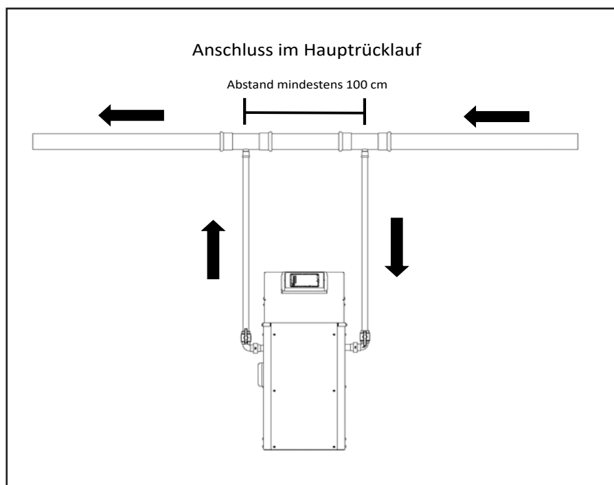
Bild 7-2: Anschlusschema Bypass-Verfahren
