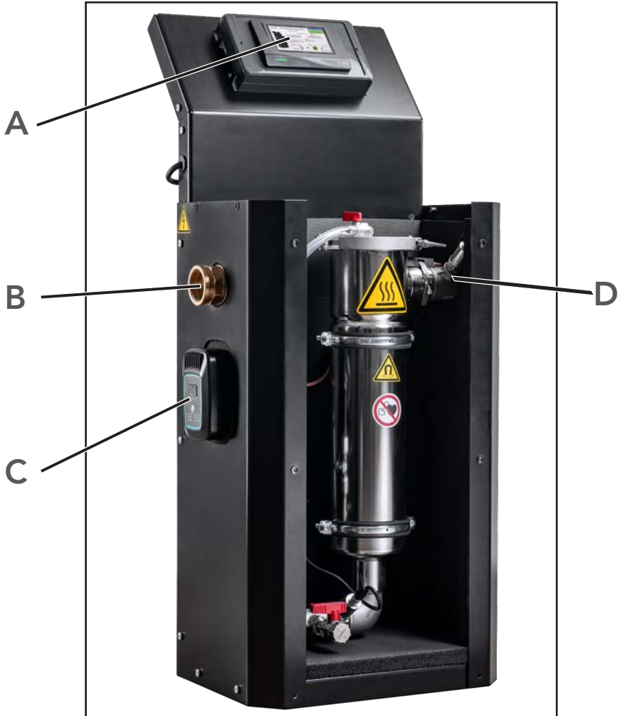
Bild 3-1: Überblick über die Bestandteile des Side Stream Filters
