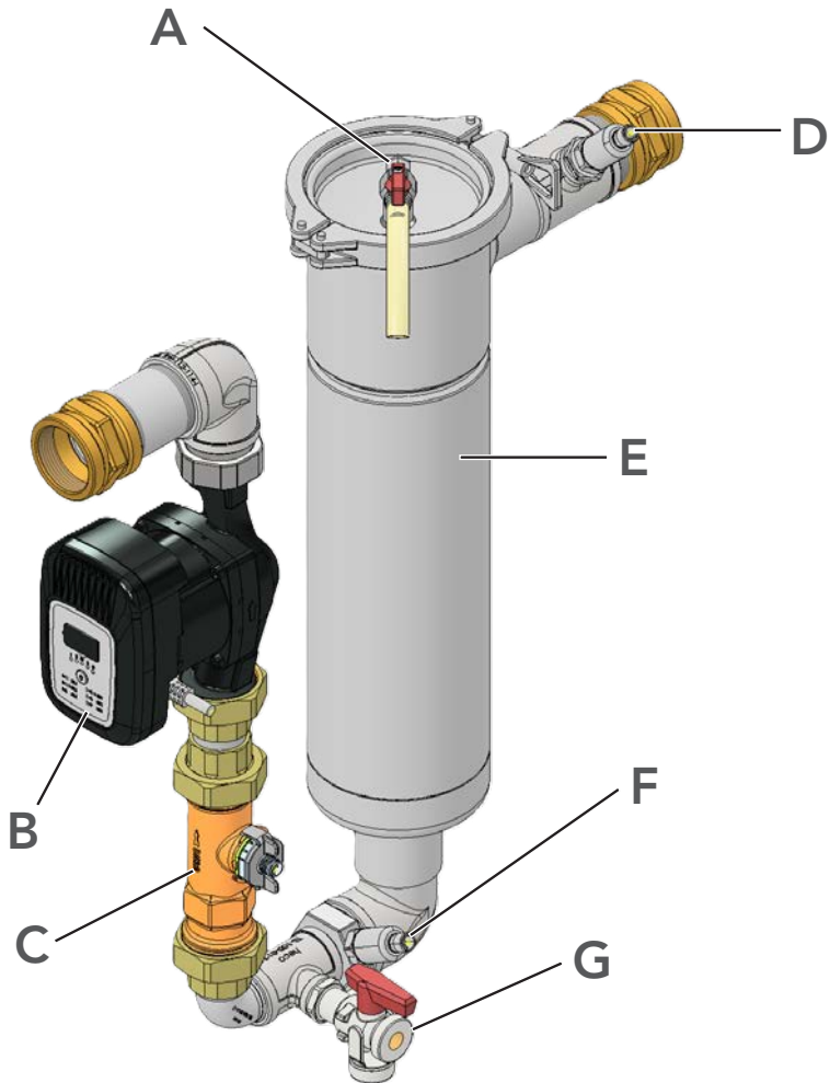
Bild 3-2: Überblick über die Komponenten des Side Stream Filters
